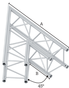
2 way corner 45°
