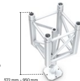
4CF30H-LEG572-950
