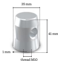
CON323
