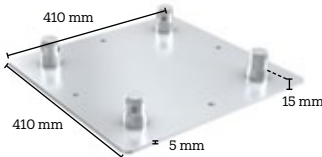
4CF30-WPC
