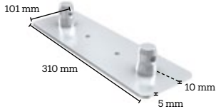
2CF30-WPC
