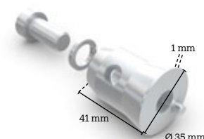
CON337
