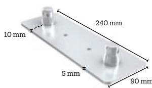
2CM22-WPC
