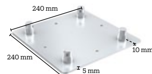
4CM22-WPC
