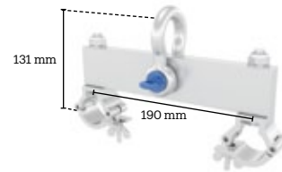
CM22-CS
