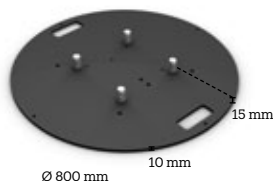
CM/CF-BP-STEEL-d800
